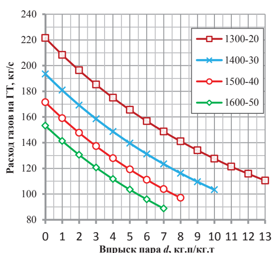
Рис. 9. Расход газов на газовую турбину в зависимости от относительного расхода пара, температуры газопаровой смеси за камерой сгорания и степени сжатия в компрессоре
