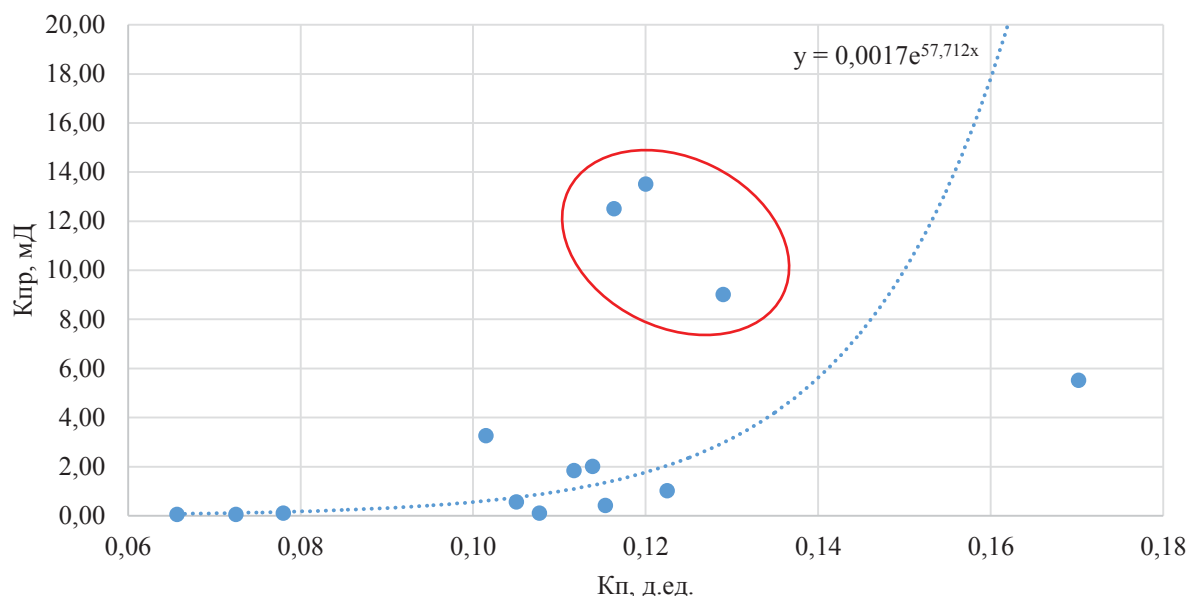
Рис. 3. Обобщенная зависимость фильтрационно-емкостных параметров нижней группы пластов ТП 19-20 танопчинской свиты
