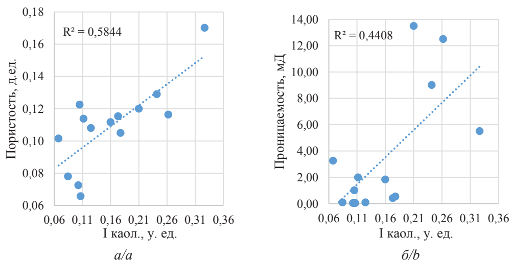
Рис. 4. График зависимости средних значений пористости (а) и проницаемости (б) от интенсивности каолинитизации нижней группы пластов ТП 19-20 танопчинской свиты
