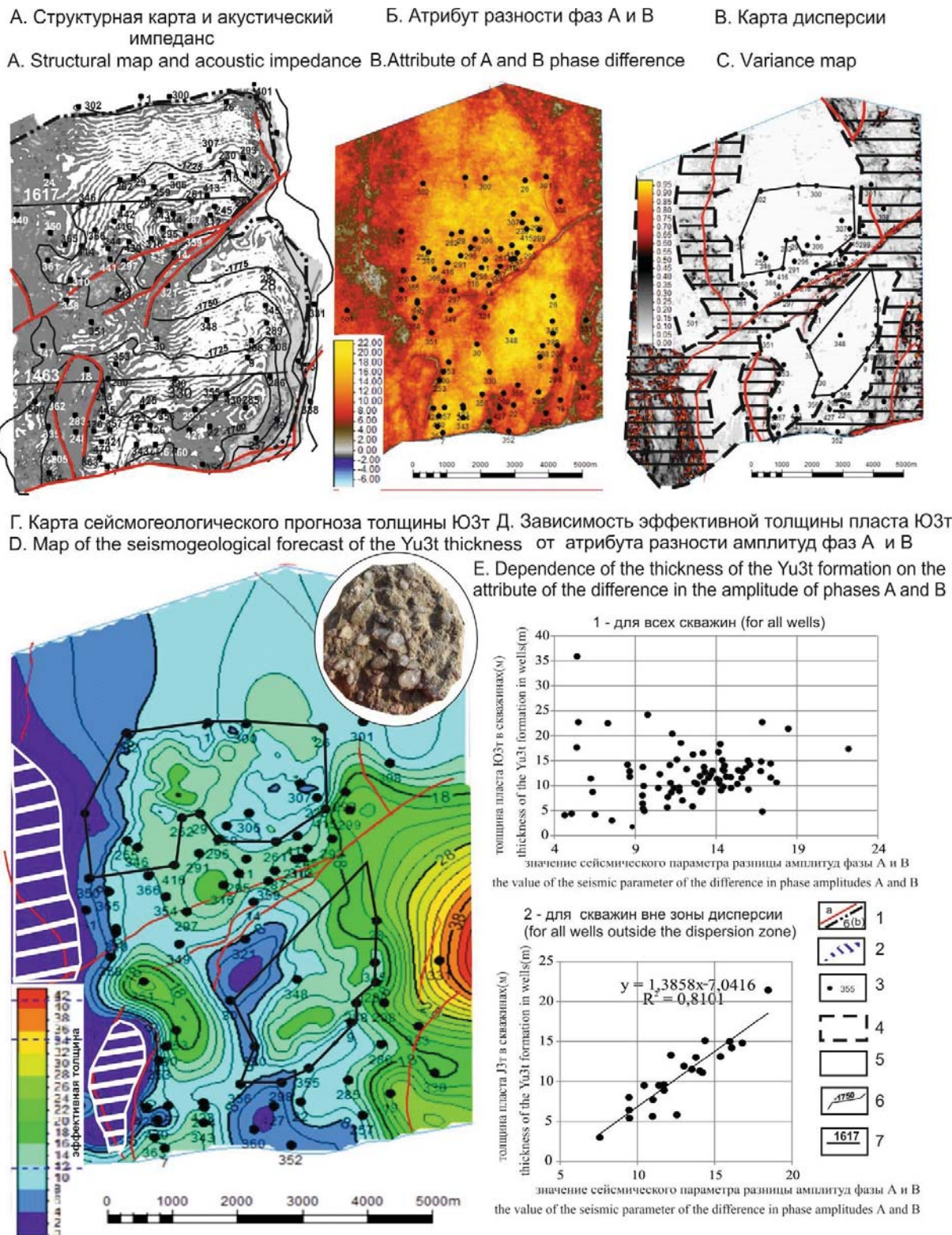
Рис. 1. Сейсмогеологический прогноз эффективной толщины пласта ЮЗт (1 – тектонические нарушения (а) и внешний контур нефтеносности (б); 2 – области выклинивания коллектора на эрозионную поверхность фундамента; 3 – скважины; 4 – тектоно-палеогеоморфологические зоны искажения динамики фазового пакета А-С; 5 – полигоны сейсмогеологического прогноза толщины пласта ЮЗт; 6 – изогипсы кровли пласта ЮЗт; 7 – сейсмические профили)
