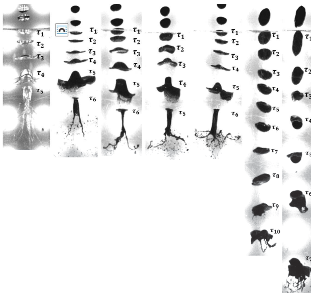
Рис. 2. Типичные кадры процесса диспергирования капель воды (а) и ВУТ (b–j). Соотношение в системе уголь/вода: а – 0/100; b – 10/90; c – 20/80; d – 30/70; e – 40/60; f – 50/50; j – 55/45 Fig. 2. Typical frames of dispersion of water droplets (a) and coal-water slurry (b–j). Ratio in the coal/water system: a – 0/100; b – 10/90; c – 20/80; d – 30/70; e – 40/60; f – 50/50; j – 55/45
