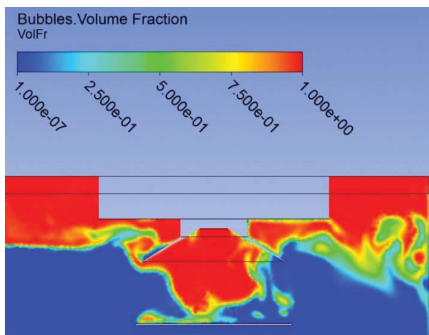
Рис. 9. Объёмная доля дымовых газов в области возле погружной горелки ( \theta=120^\circ )
