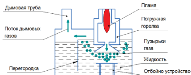
Рис. 1. Принципиальная схема лабораторной установки Fig. 1. Schematic diagram of a laboratory setup
