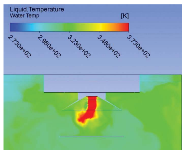
Рис. 7. Температура жидкости в области возле погружной горелки ( \theta=120 с)
