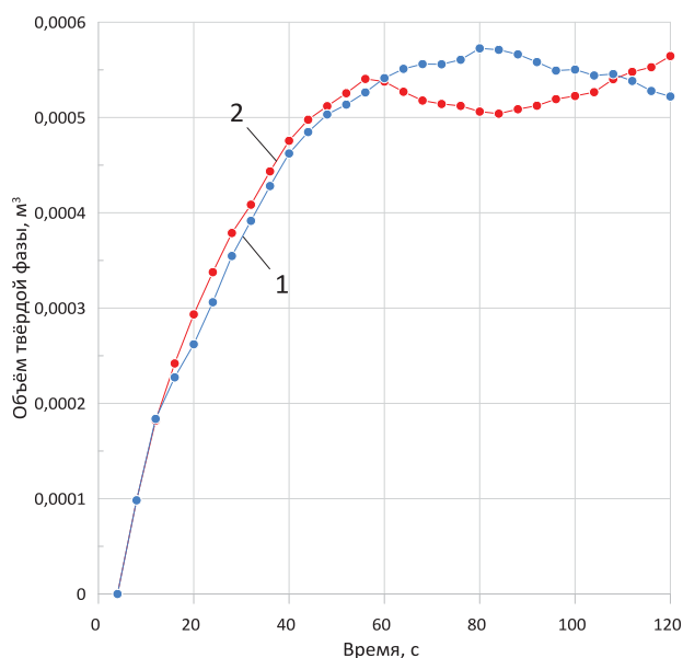
Рис. 5. Объём твёрдой фазы, распределённой в жидкости: 1 – сток 0,1 кг/с; 2 – сток 1 кг/с
