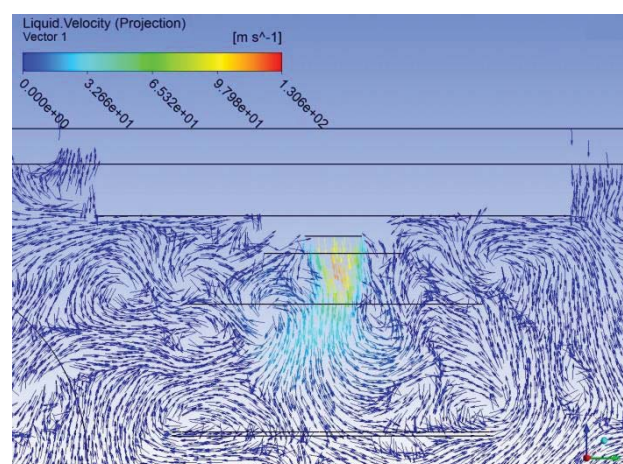
Рис. 8. Скорость жидкости в области возле погружной горелки ( \theta=120 с)
