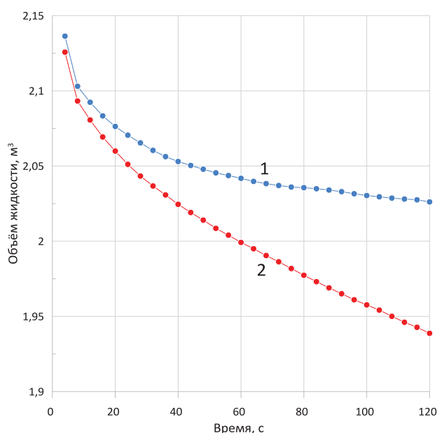
Рис. 6. Объём жидкости: 1 – сток 0,1 кг/с; 2 – сток 1 кг/с
