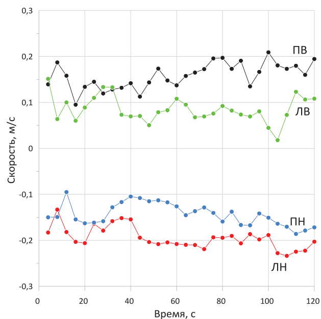
Рис. 11. Проекция скорости жидкости на ось X: ПН – правая нижняя точка; ЛН – левая нижняя точка; ЛВ – левая верхняя точка; ПВ – правая верхняя точка
