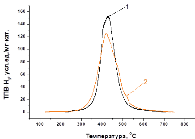
Рис. 6. Кривые ТПВ-H 2 для катализаторов, модифицированных барием: 1 – Cr(3 %)O x /КСКГ; 2 – Cr(3 %) O x /PA (20) – Ba/КСКГ
