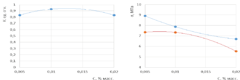
Рис. 9. Влияние содержания сульфонола (C) на водостойкость (K, ед. отн.) и на прочность (σ, МПа) ангидритовых образцов
