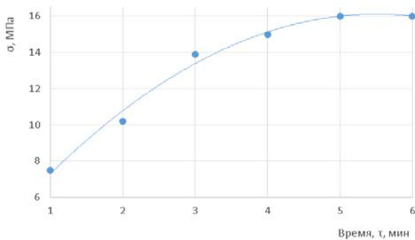
Рис. 5. Влияние времени перемешивания ( \tau , мин) ангидритового раствора на предел прочности сжатию ( \sigma , МПа)
