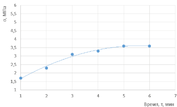
Рис. 6. Влияние времени перемешивания ( \tau , мин) ангидритового раствора на предел прочности изгибу ( \sigma , МПа)
