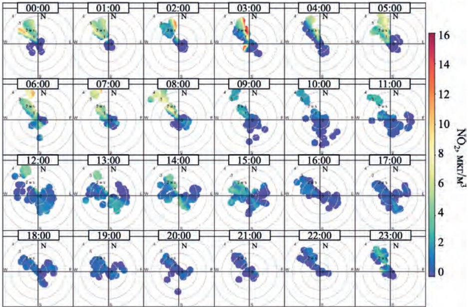
Рис.4. NWR-анализ для десятиминутных концентраций NO 2 в полярной системе координат на ст. «Листвянка», июль 2023 г
