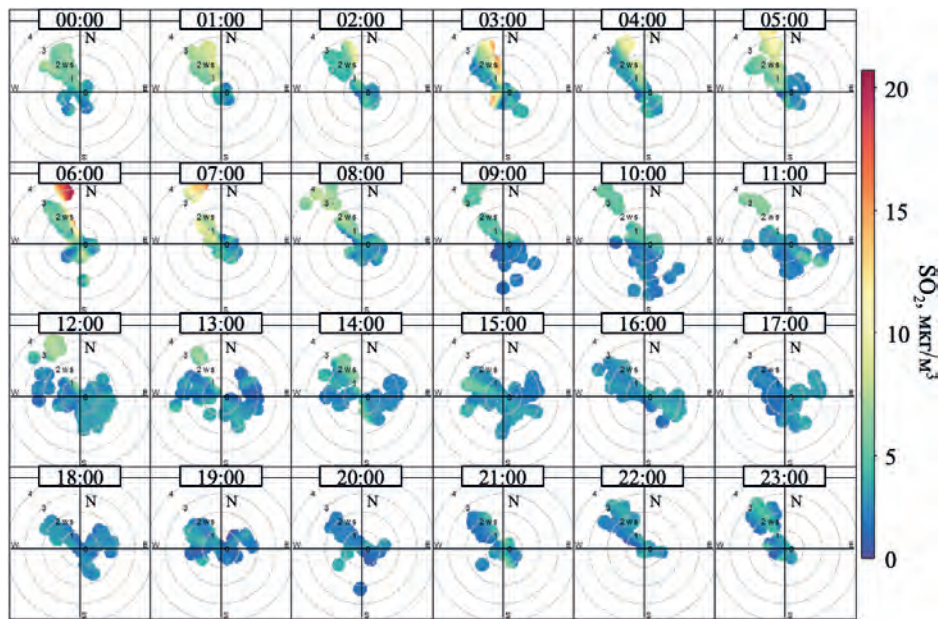
Рис.3. NWR-анализ для десятиминутных концентраций \text{SO}_2 в полярной системе координат на ст. «Листвянка», июль 2023 г.
