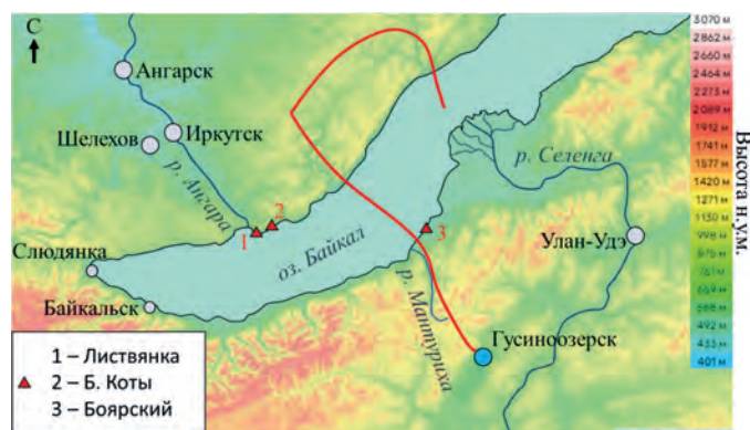
Рис.9. Топографическая карта исследуемого региона ( https://ru-ru.topographic-map.com ) и прямая траектория движения воздушных масс от стационарных источников г. Гусиноозерск на высоте 500 м AGL, 20.07.2023 7:00 МВ.
