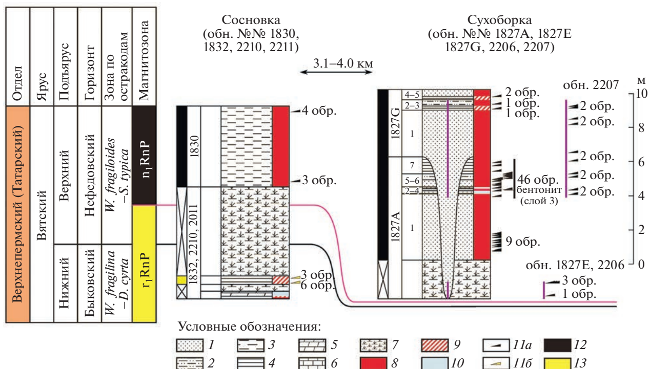
Рис. 1. Интервалы опробования разрезов Сухоборка и Сосновка и количество отобранных образцов. Номера обозначений даны (по В.К. Голубеву). Условные обозначения: 1 – песок; 2 – алеврит песчаный; 3 – алеврит глинистый; 4 – глина; 5 – мергель; 6 – известняк; 7 – осыпь; 8 – красноцветы; 9 – пестроцветы; 10 – сероцветы; 11 – уровни отбора палеомагнитных образцов с характеристической компонентой ЕОН: прямой полярности (а), обратной полярности (б); 12 – зоны прямой (N) полярности; 13 – зоны обратной (R) полярности.
