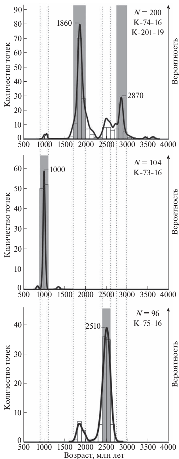
Рис. 4. Распределение возраста зерен циркона на гистограммах и кривых относительной вероятности для песчаников деревнинской свиты (обр. K75/16), трахита (обр. K73/16) и шамозитовых песчаников (обр. K74/16, K201/19) нижнетунгусской свиты.
