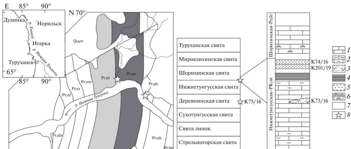
Рис. 1. Геологическая схема позднего докембрия Туруханского поднятия и фрагмент литологической колонки верхней части нижнетунгусской свиты и нижней части шорихинской свиты. 1 – известняк, 2 – глинистый известняк, 3 – трахит, 4 – бедные бокситовые руды, 5 – шамозиты, 6 – строматолитовые известняки, 7 – перерыв в наблюдениях, 8 – место отбора проб на U–Pb-датирование циркона. Свиты Туруханского поднятия: Pr 3 ln – линок, Pr 3 sh – сухотунгусская, Pr 3 dr – деревнинская, Pr 3 nt – нижнетунгусская, Pr 3 sr – шорихинская, Pr 3 mr – мироедихинская, Pr 3 tr – туруханская, Pr 3 dm – дурномысская; Q IIIsg – четвертичные отложения.
