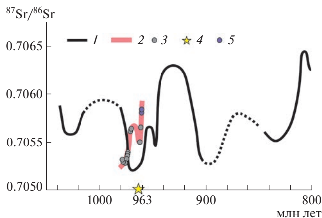
Рис. 6. Сопоставление данных Sr-хемостратиграфии для раннепротерозойских карбонатных пород. 1 – кривая вариаций изотопного состава Sr в воде раннепротерозойского океана [2, 3], 2 – фрагмент уточненной кривой вариаций состава Sr в воде ран-непротерозойского океана на основе данных, полученных в данной работе, 3 – значения ^{87}\text{Sr}/^{86}\text{Sr} в карбонатных породах верхней части нижнетунгусской свиты, 4 – возраст вулканитов, синхронных с накоплением карбонатных отложений нижнетунгусской свиты, 5 – значения ^{87}\text{Sr}/^{86}\text{Sr} в карбонатных отложениях основания шорихинской свиты.
