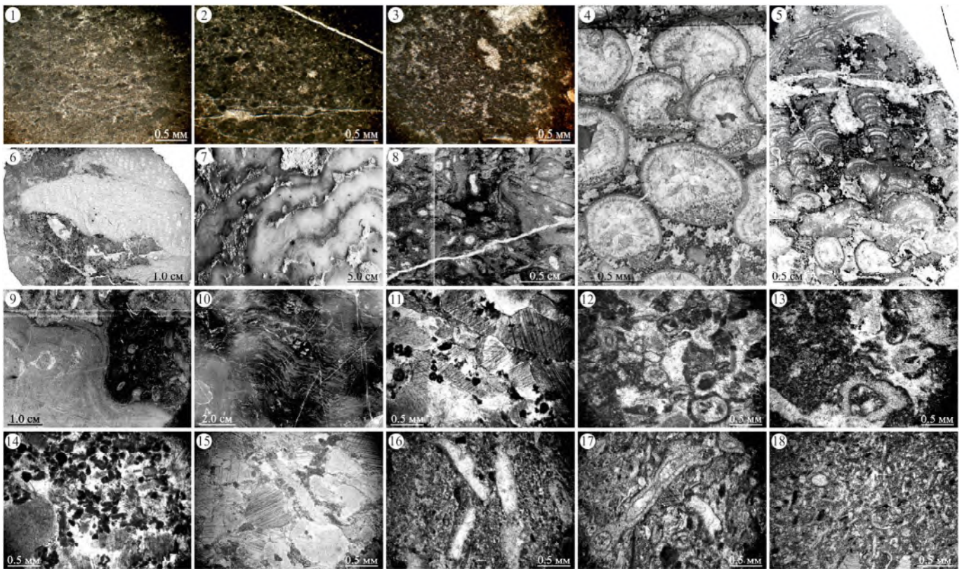
Рис. 4. Литологические типы биохемотрогенной, биогенной и механогенной (подгруппа биокластовых известняков) групп верхнеордовикских карбонатных отложений шежимского фациального комплекса: 1—3 — известняки биохемотрогенные: 1 — пелитоморфный (ЛТ-1), 2 — микрокомковатый (ЛТ-2), 3 — микросгустковый (ЛТ-3); 4—10 — известняки биогенные: 4 — биогермный цианобактериально-губковый доломитистый (ЛТ-4), 5 — биогермный губково-водорослевый (ЛТ-5), 6 — биогермный водорослево-коралловый (ЛТ-6), 7 — биогермный водорослево-строматопороидный (ЛТ-7), 8 — биогермный гидроидный доломитистый (ЛТ-8), 9 — биогермный водорослевый (ЛТ-9), 10 — биогермный строматолитовый (ЛТ-10); 11—17 — известняки механогенные, грубо- и крупнобиокластовые: 11 — цианобактериально-криноидный (ЛТ-11), 12 — водорослево-криноидный (ЛТ-12), 13 — участок темно-серого сгусткового известняка с пятнистой доломитизацией в водорослево-криноидном известняке (ЛТ-12), 14 — микрокомковато-криноидный (ЛТ-13), 15 — криноидный (ЛТ-14), 16 — гидроидный (ЛТ-15), 17 — водорослевый (ЛТ-16); 18 — известняк механогенный микробиокластовый (ЛТ-17)
