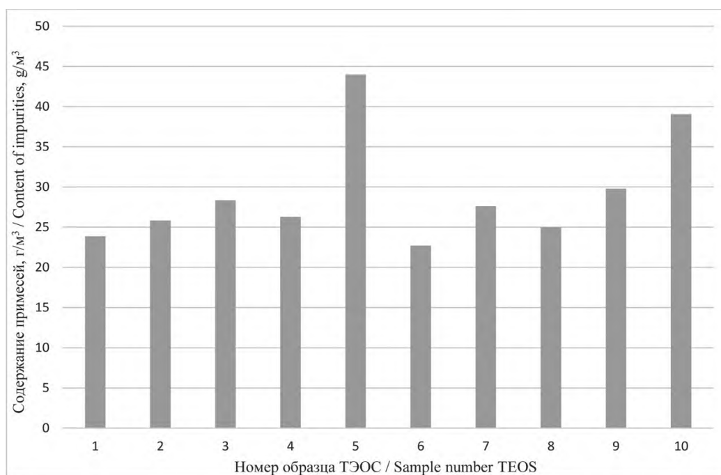
Рис. 3. Общее содержание элементов-примесей (г/м³) для системы C_2H_5OH-NH_4OH-H_2O-SiO_2 с использованием тетраэтоксисилана различных производителей (в соответствии с табл. 1)
