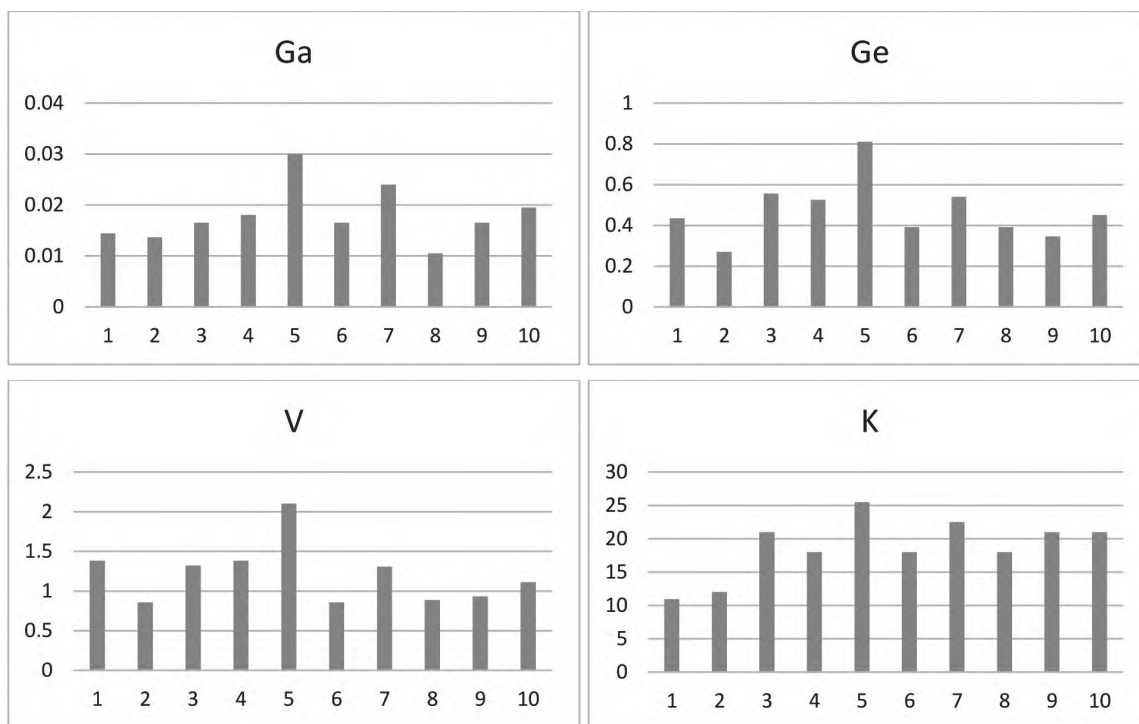
Рис. 2. Содержание элементов-примесей Ga, Ge, V, K (г/м³) для системы C_2H_5OH-NH_4OH-H_2O-SiO_2 с использованием тетраэтоксисилана различных производителей (в соответствии с табл. 1) (ось X)
