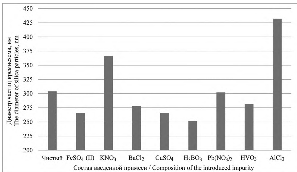
Рис. 4. Зависимость размеров сформировавшихся в результате гидролиза монодисперсных сферических частиц кремнезема от типа введенной в исходный этиловый спирт примеси в сравнении с синтезом, проведенным без добавок
