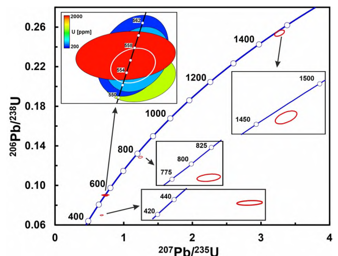
Рис. 7. Диаграмма с конкордией для кристаллов циркона из гранитов скв. 11-Малая Пера. Конкордантный возраст 557 \pm 1 млн лет ( 2\sigma , n = 8 , CKBO = 1.5 )
